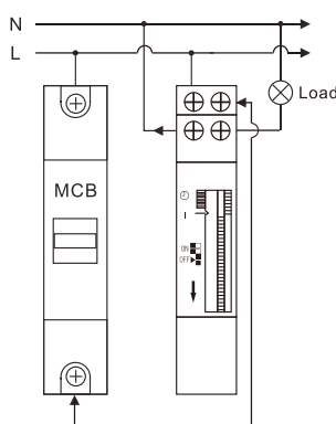
wiring diagram:
