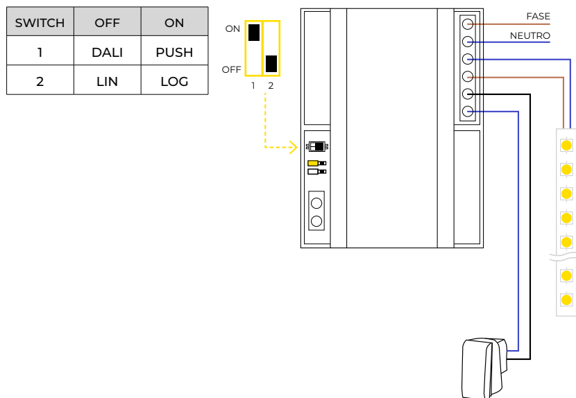
FIG. 3 - Schema collegamento 6 fili (consigliato)
