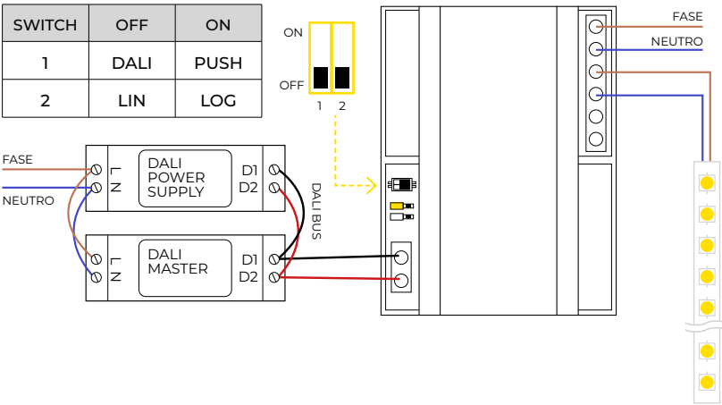
FIG. 1 - Schema collegamento 4 fili (consigliato)
