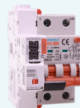
Wi-Fi + RIARMO AUTOMATICO 2P · 3M
