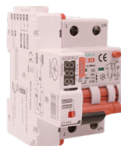
RIARMO AUTOMATICO 2P · 3M · 3 tentativi
