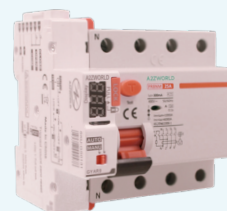
PR8NM · RIARMO AUTOMATICO / Wi-Fi
