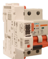
RIARMO AUTOMATICO 2P · 3M · 3 tentativi
